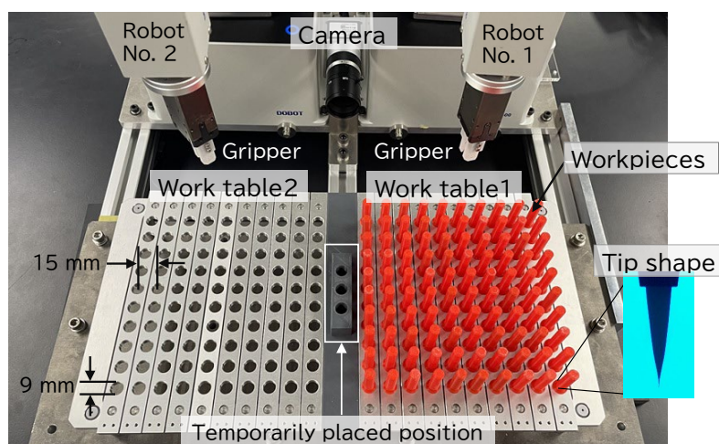
図 複数ロボットの協調動作による化粧用具の不良品の自動分別
