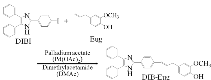
図 1 DIBI によるオイゲノールの蛍光誘導体化反応
